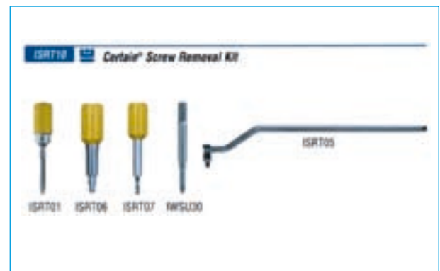
Afb. 4. Hulpset voor verwijdering van een gefractureerde implantaatopbouwsschroef van het Osseotite®-systeem met boorgeleidend instrumentarium voor een implantaat met een interne connectie.
