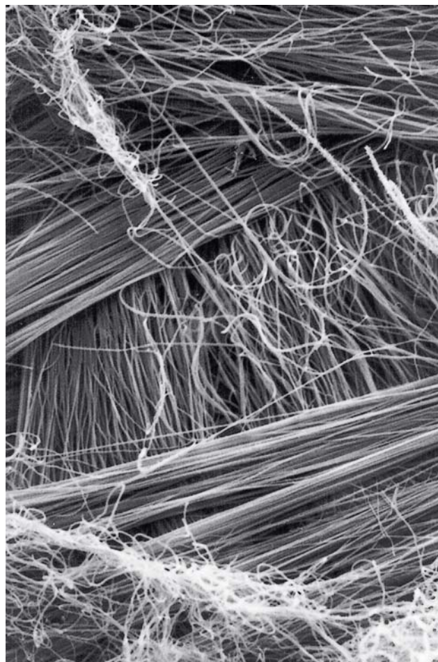
Afb. 2. Opname met scanningelektronenmicroscopie van het oppervlak van het caput mandibulae. De collageenefibrillen vormen een duidelijk vlechtwerk ( \times 4.000 ).
