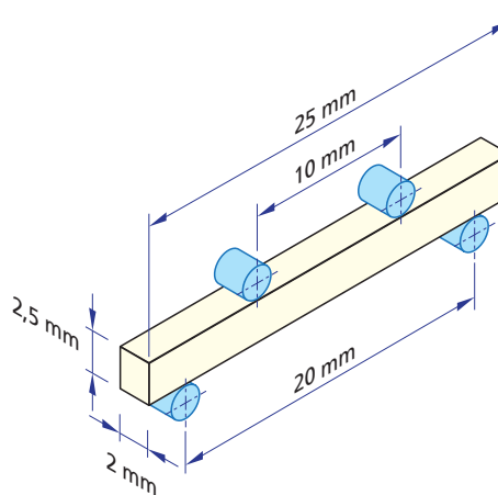
Afb. Vierpuntenbuigtest.
