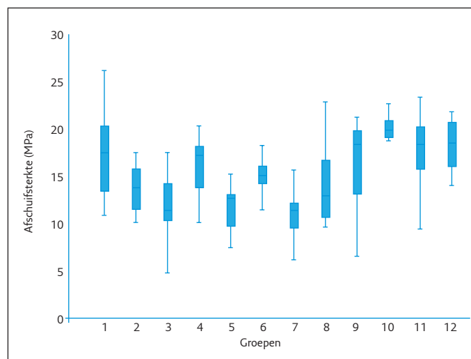
Afb. 2. Afschuifsterkte van composiet gehecht aan composiet (MPa).
